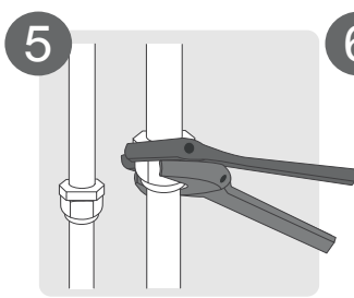
5 Подключите трубопроводы
