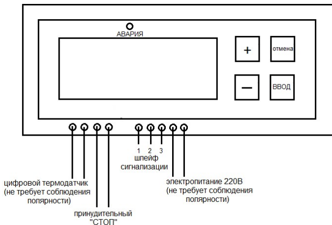
Схема электроподключения на рис 1.
